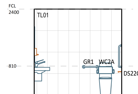
6 ELEVATION DETAIL 60-130 1 : 50
